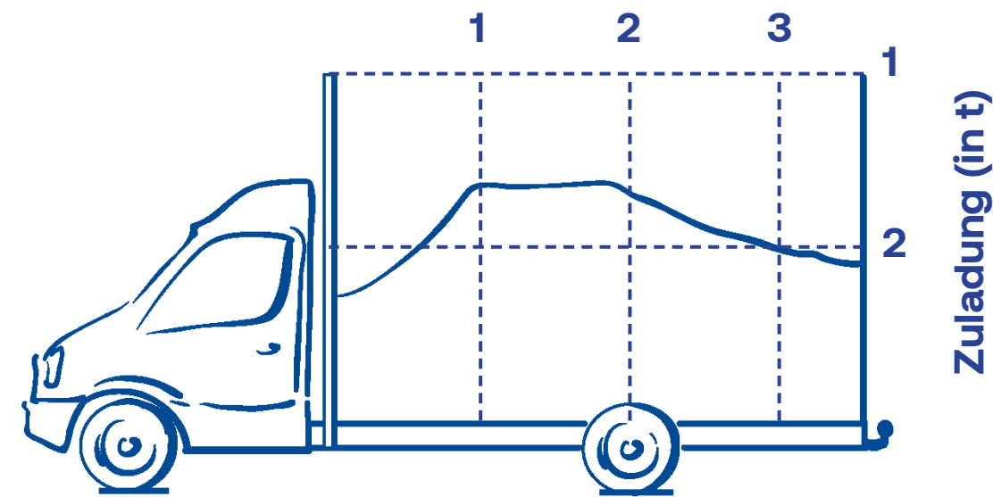
Korrekte Verteilung
