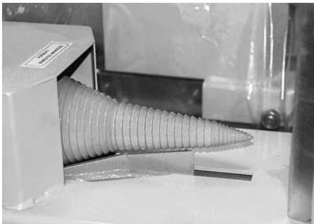
Bild 29 Spaltkeil und Zuführvorrichtung
