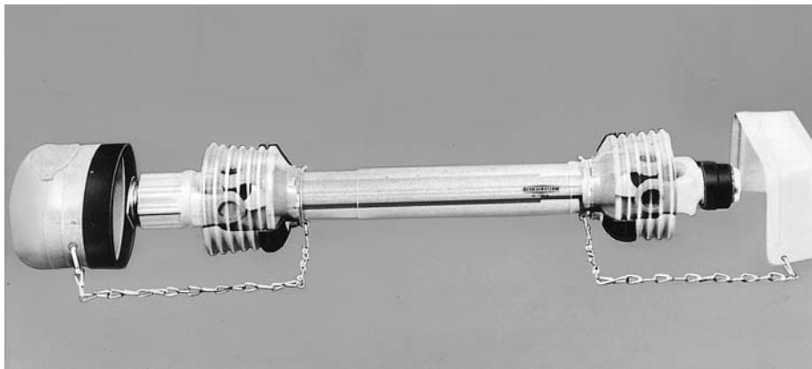
Bild 3 Verdeckte Gelenkwelle zwischen Antriebsaggregat und Anbaugerät.
