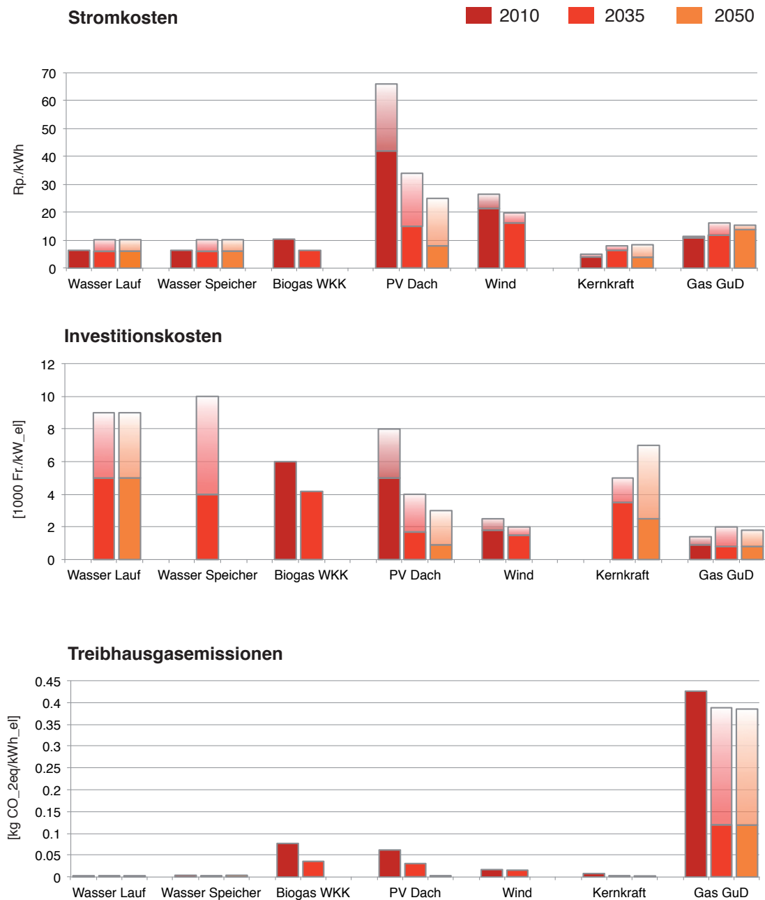
Abbildung 3: Vergleich von ausgewählten Stromproduktionsarten unter den Gesichtspunkten Stromkosten, Investitionskosten und Treibhausgasemissionen für die Jahre 2010, 2035 und 2050. Die helleren Schattierungen geben die Bandbreite an. Die heutigen und erwarteten Stromkosten, Investitionskosten und Treibhausgasemissionen der wichtigsten Stromproduktionsarten in der Schweiz basieren auf Lebenszyklusanalysen. Die tiefen Emissionswerte der GuD ab 2035 und entsprechend höheren Kosten schliessen die CO 2 -Abscheidung und Speicherung mit ein. Die Zahlen einer einzelnen Anlage können von diesen Werten stark abweichen, je nach Standort, Auslastung, Lebensdauer und Verzinsung oder aufgrund von Bauverzögerungen. Jede Produktionsart hat zudem ganz spezifische Produktionscharakteristiken. Während der Stromverbrauch im Winter am höchsten ist, produzieren die Wasserkraft und die Photovoltaik im Sommer am meisten Strom. Die Elektrizität aus Photovoltaik und Windkraft fällt fluktuierend an. Je nach Anlagentyp sind zudem weitere Anlagen erforderlich wie Speicher oder Stromleitungen. (Datenquelle: Hirschberg 2010)
